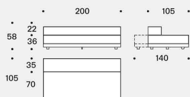
Divano - letto / Sofa - bed
